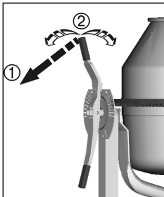
nastavitveni vzvod
